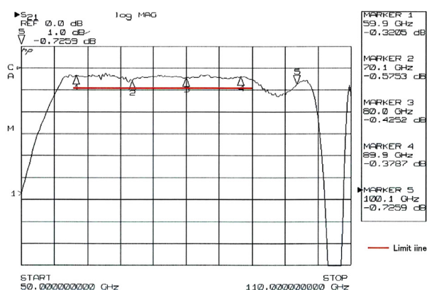
挿入損失
