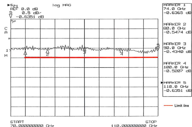
挿入損失
