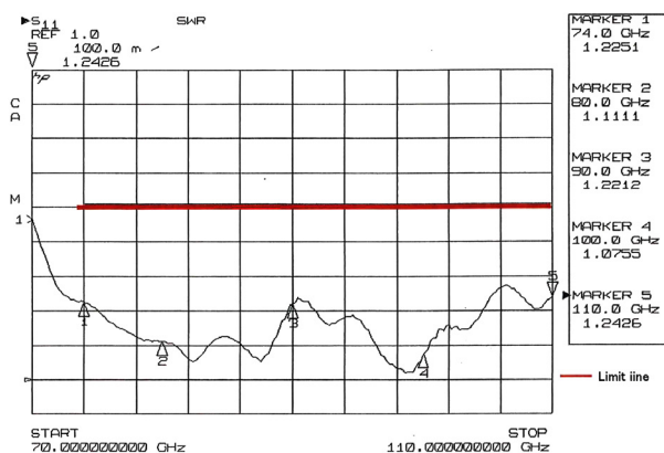
VSWR
