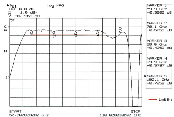
挿入損失
